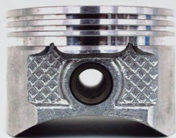
PISTÓN STD PARA COMPRESOR 904
