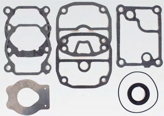
REPUESTO MAYOR PARA COMPRESOR KNORR 190 (059-F)
