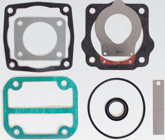
REPUESTO PARA COMPRESOR KNORR 150
