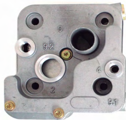
CABEZA ARMADA DE COMPRESOR 906
